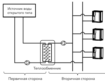
Водяной контур открытого типа с теплообменником
