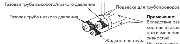
Для системы регенерации тепла Фиксация жидкостных труб, газовых труб низкого давления и газовых труб высокого/низкого давления
