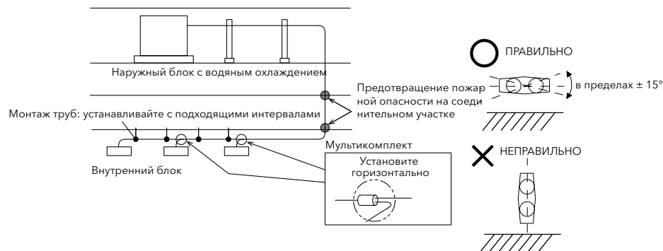
Пример фиксации труб
