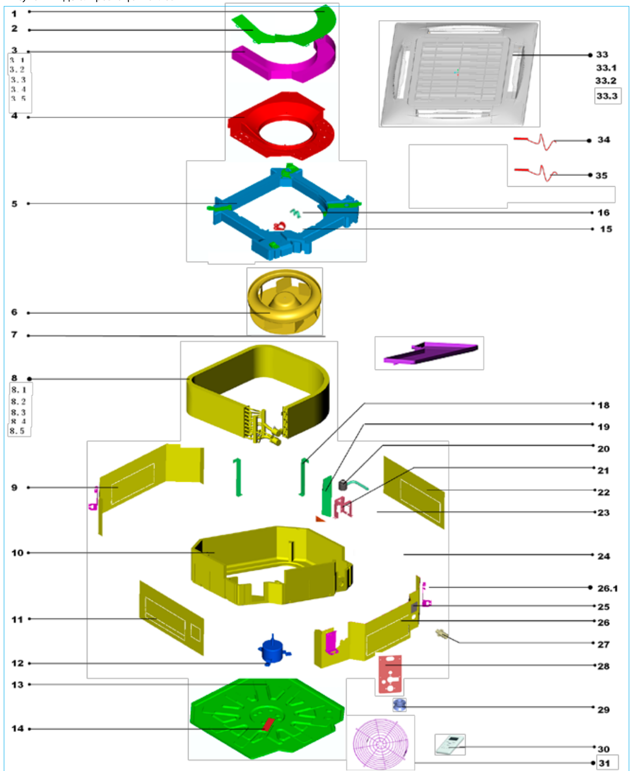
Рисунок №7 Детализовка фанкойлов
