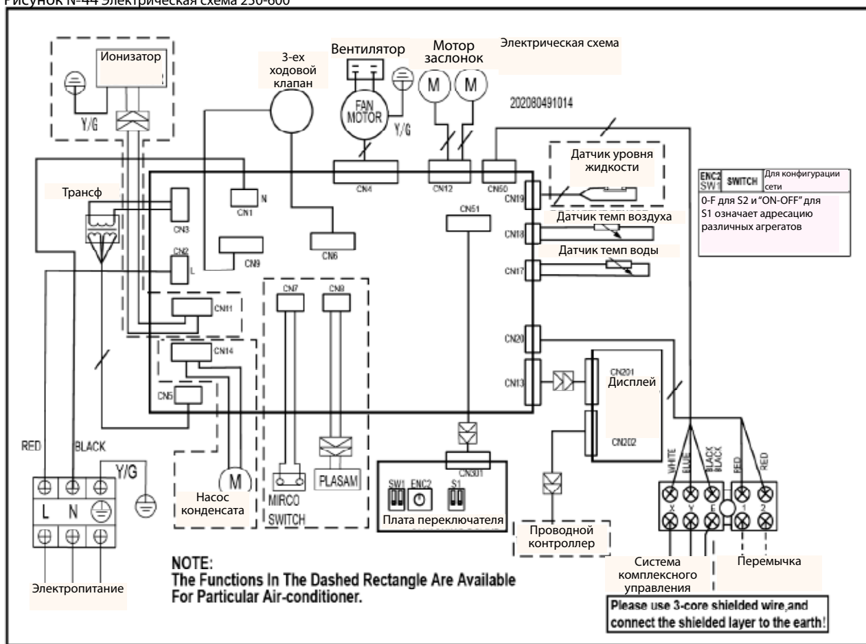
Рисунок №44 Электрическая схема 250-600
