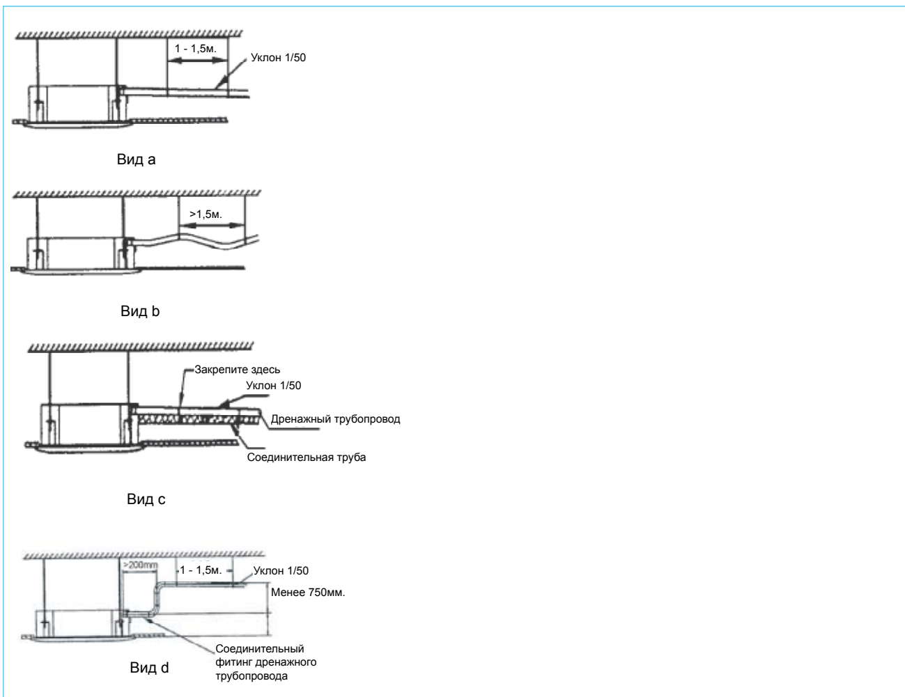
Рисунок №23 Монтаж дренажного трубопровода
