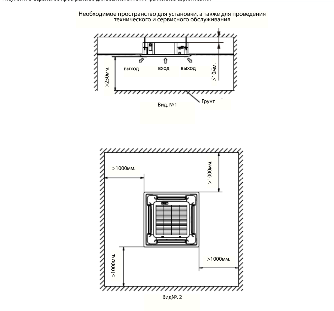
Рисунок №3 Сервисное пространство для всех исполнений фанкойлов серии M(D)КА
