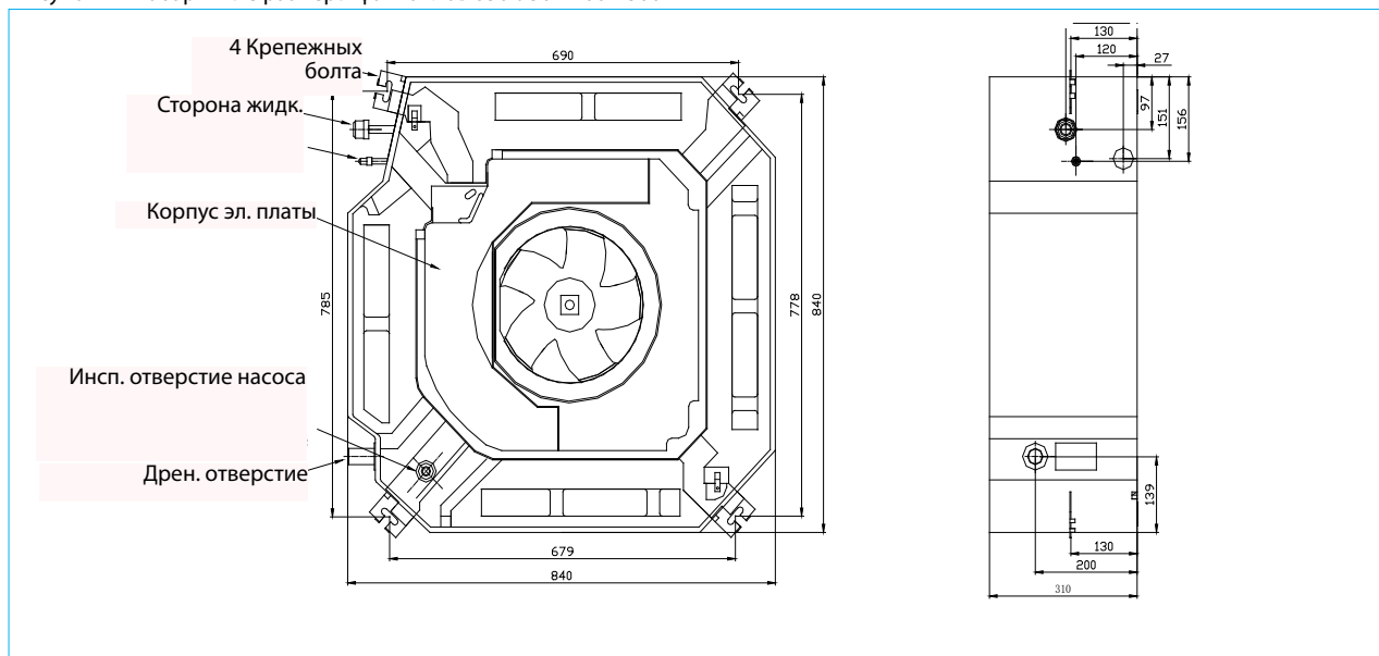
Рисунок №2 Габаритные размеры фанкойлов 850-950-1200-1500
