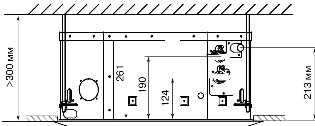
Рисунок №14 Пространство, необходимое для возможного ремонта и технического обслуживания
