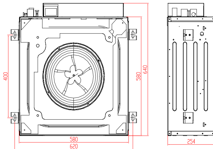
Рисунок №13 Габаритные размеры фанкойлов
