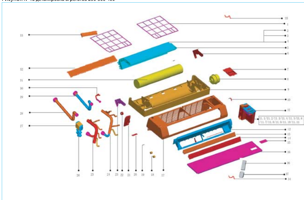
Рисунок №46 детализовка агрегатов 250-300-400
