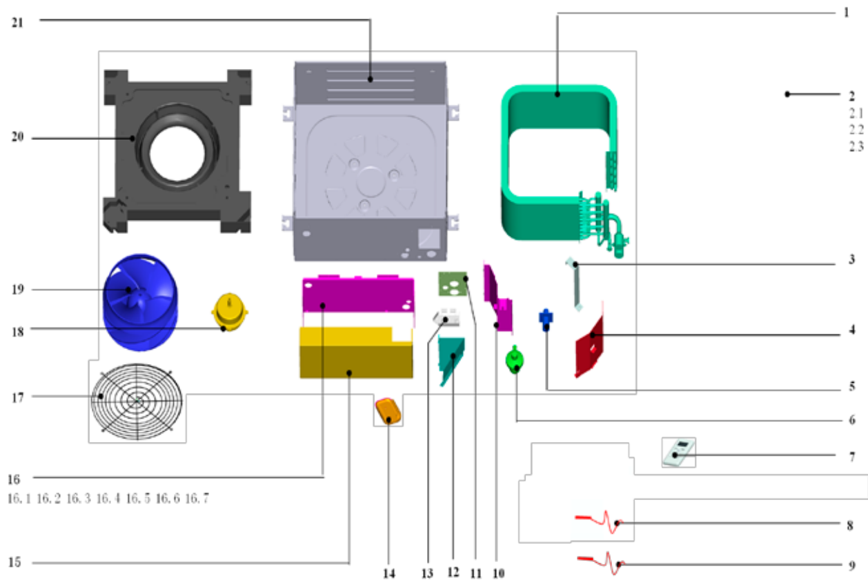
Рисунок №18 Детализовка агрегатов
