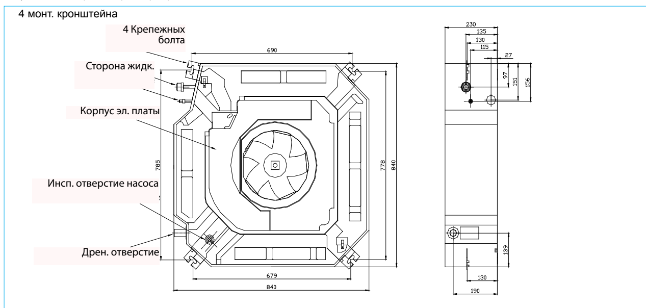
Рисунок №1 Габаритные размеры фанкойлов 600-750
