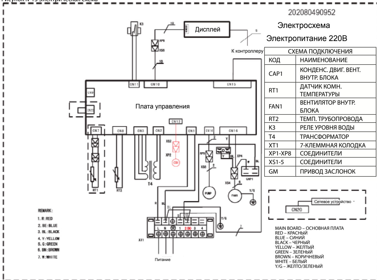
Рисунок №15 Электрическая схема
