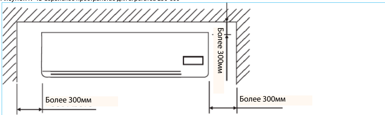
Рисунок №43 Сервисное пространство для агрегатов 250-600
