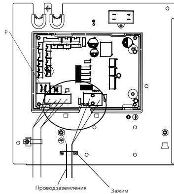
Увеличенный вид проводниклеммной коробки(ТВ), деталь P
